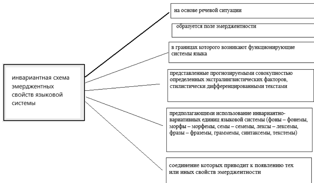
Рис. 1. Инвариантная схема эмерджентных свойств языковой системы.
